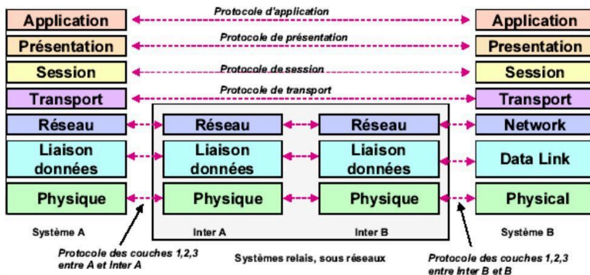
[Figure 1 : Communication impliquant un système ouvert de relais]
