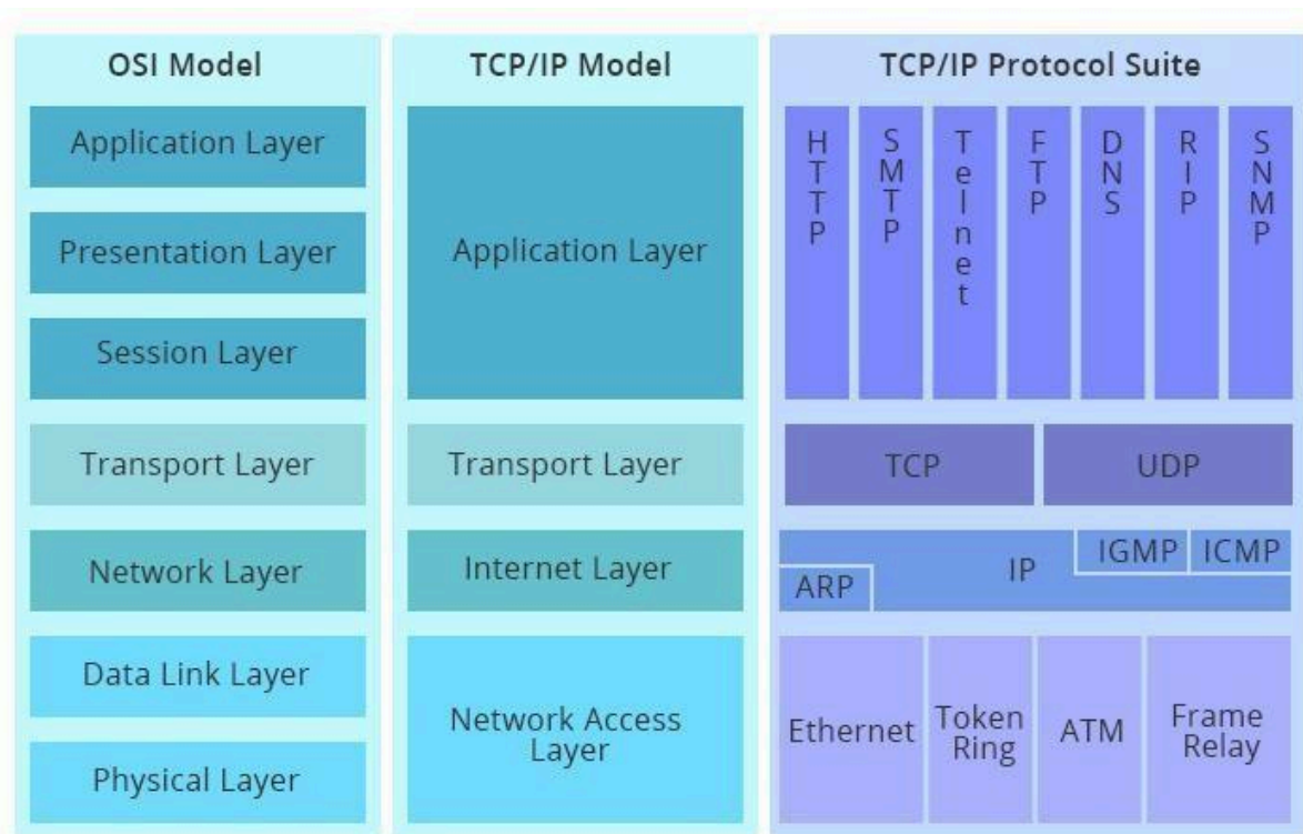
[Figure 9 : Analogie entre le modèle OSI et le modèle TCP/IP]
